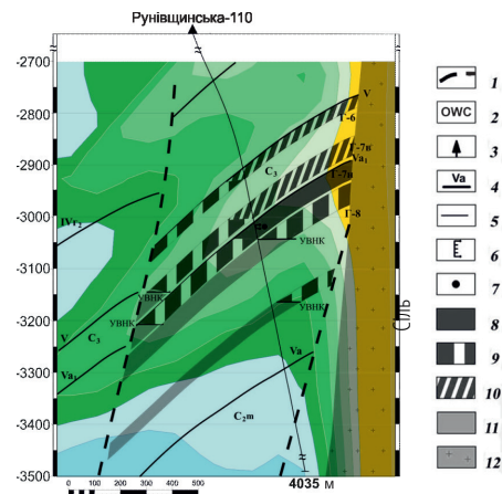
1 - тектонічні порушення, 2 - умовний водонафтовий контакт (УВНК), 3 - пошукова свердловина, 4 - сейсмічні границі, 5 - стратиграфічні границі, 6 - інтервали випробувань, 7 - приплив нафти, 8 - нафтоносний колектор, 9 - прогнозні нафтові поклади, 10 - нафтоносність за даними промислової геофізики, 11 - водоносний колектор, 12 - соляний шток
