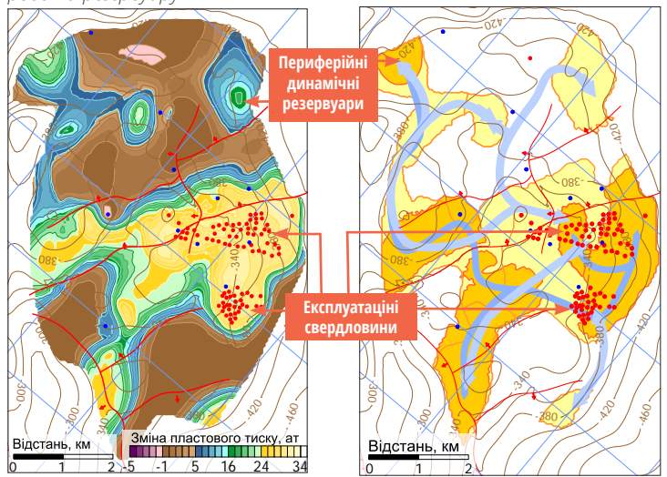
Рисунок 6. Зміна пластового тиску (ліва) і положення динамічних резервуарів та шляхів міграції газу в межах горизонту зберігання НД-8 (права)
