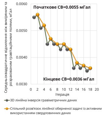
Рисунок 5. Ітеративне покращення 3D моделі густини в результаті розв'язку оберненої 3D задачі гравірозрахунку
