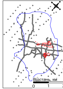
Рисунок 2. Схема розташування пунктів повторних гравіметричних спостережень
