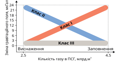
Рисунок 1. Періоди проведення повторних гравіметричних спостережень та динаміка зміни кількості газу в Дашавському ПСГ
