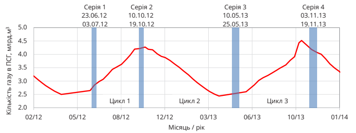
Рисунок 1. Періоди проведення повторних гравіметричних спостережень та динаміка зміни кількості газу в Дашавському ПСГ
