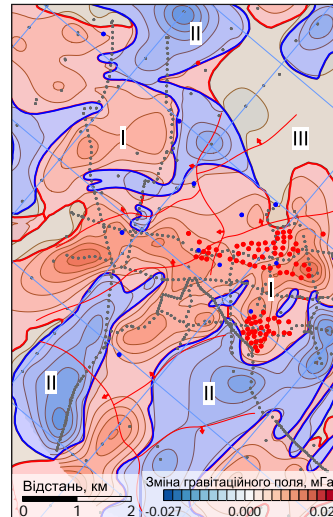
Рисунок 4. Аномальне гравітаційне поле, зумовлене закачуванням газу в ПСГ та класифікація згідно режиму роботи резервуару
